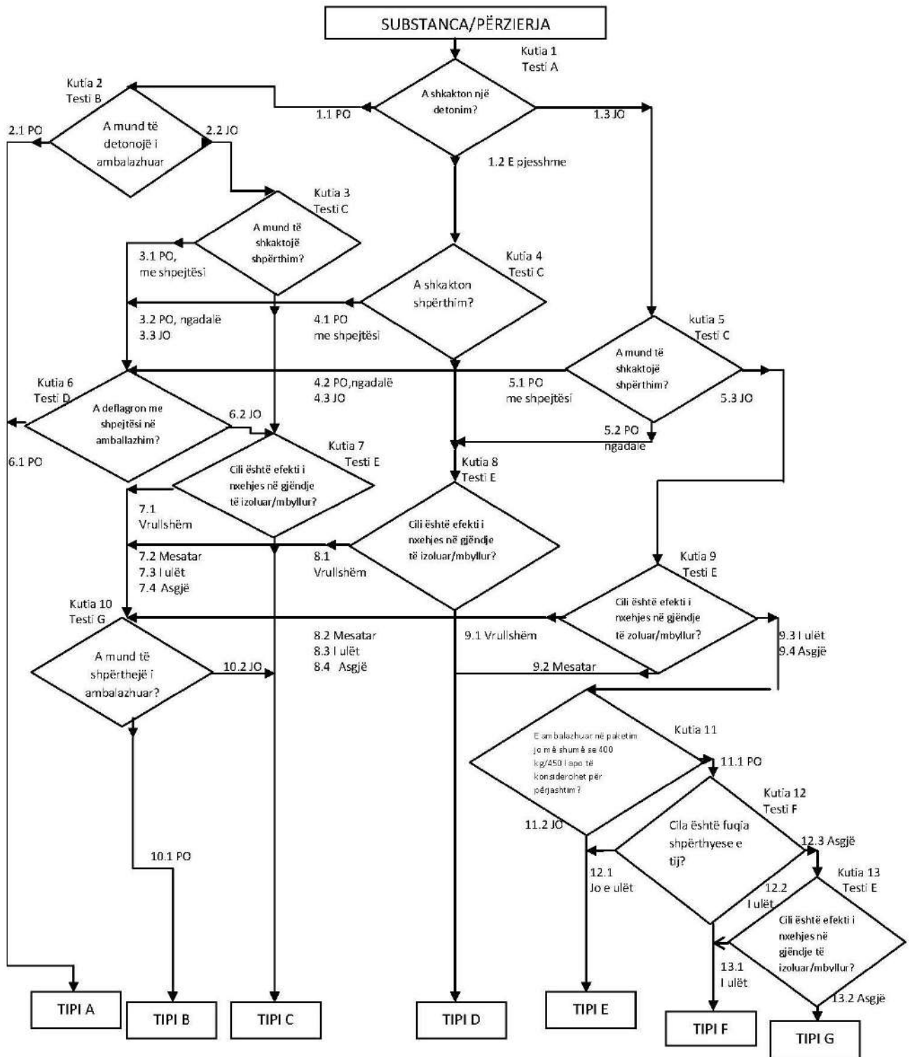
Figura 2.15.1 Peroksidet Organike
