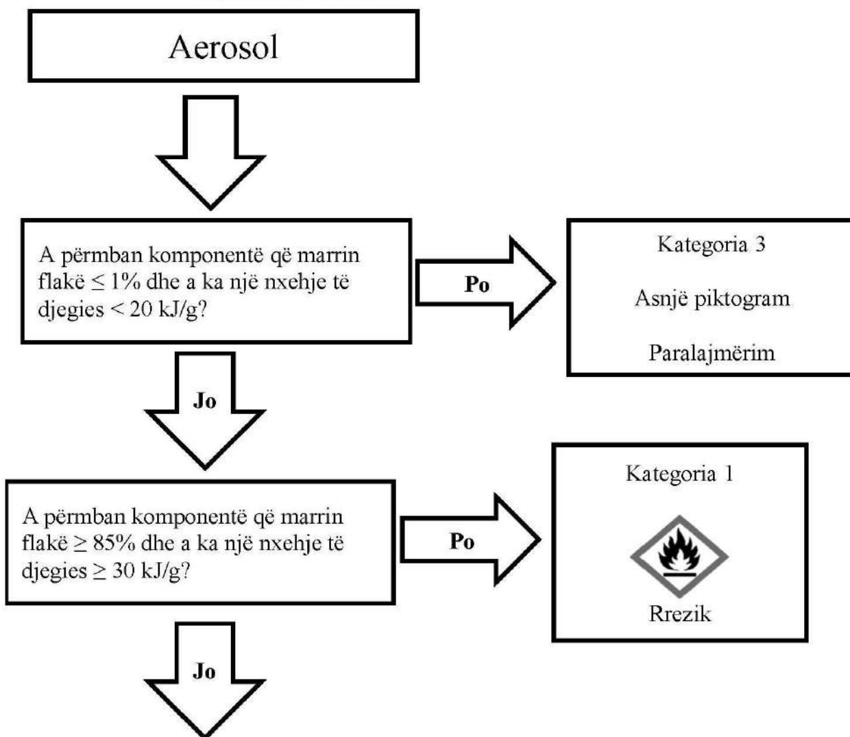
Figura 2.3.1 (a) Aerosolët
