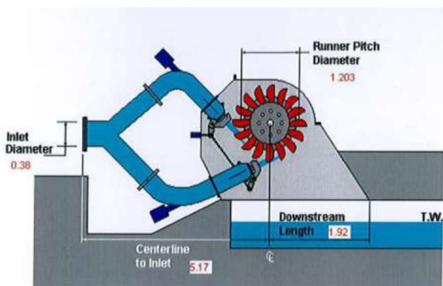
Imazh ilustrativ i Turbinave TIP te llojit Pelton
