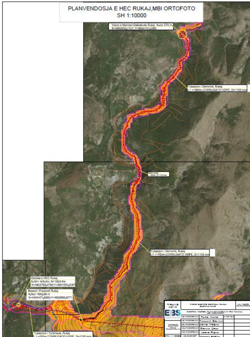
Figura 2: Planimetria e vendosjes se Hec RRUKAJ
