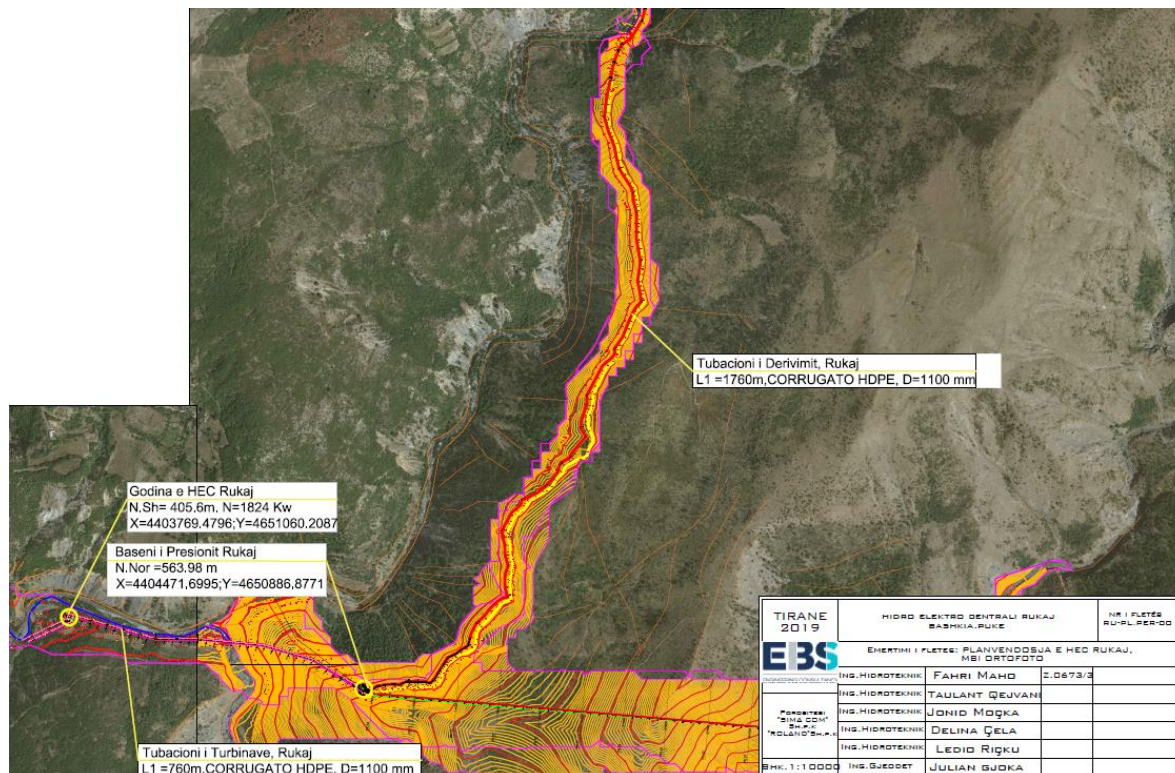
Figura 1: Planimetria e Pergjithshme e vendosjes se veprave te Hec RRUKAJ me koordinata, (vendosur bashkengjitur raportit ne format A3)
