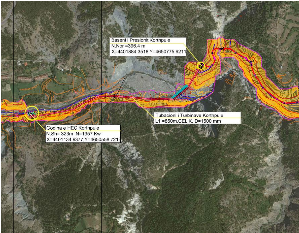
Figura 1: Planimetria e Pergjithshme e vendosjes se veprave te Hec KORTHFULA me koordinata, (vendosur bashkengjitur raportit ne format A3)
