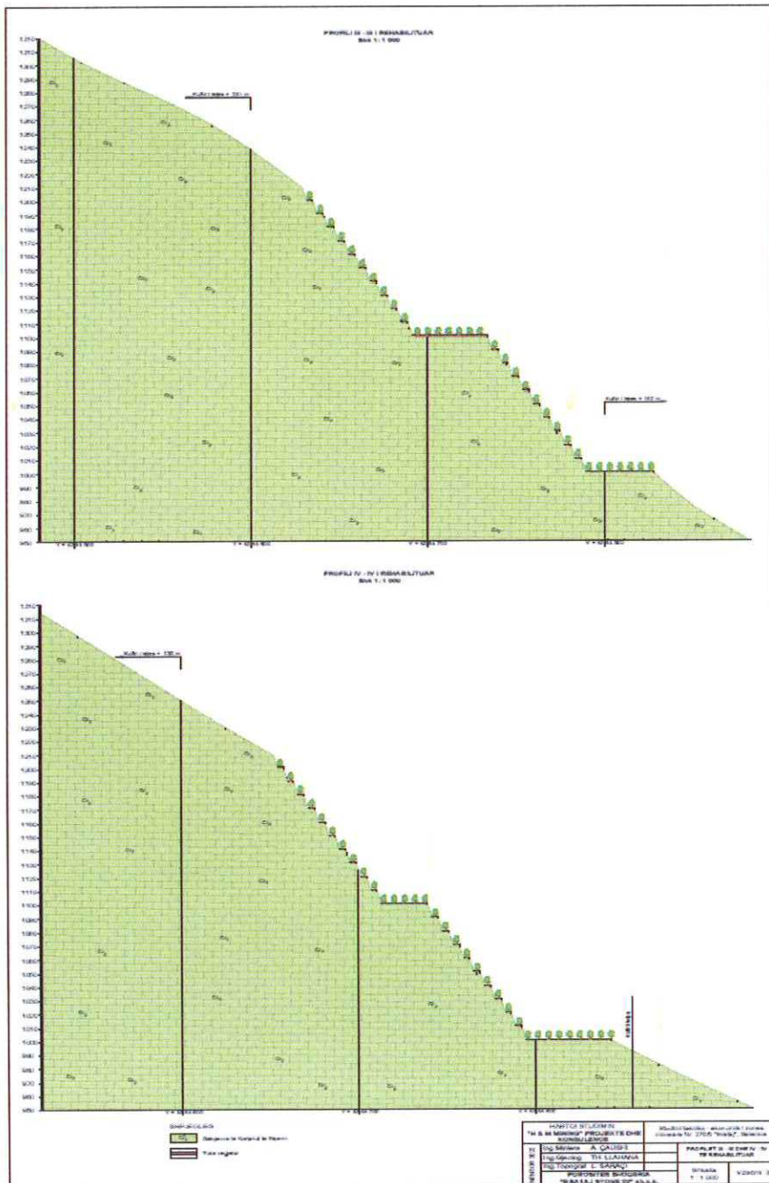
Profilet III-III dhe IV-IV te rehabilituar
