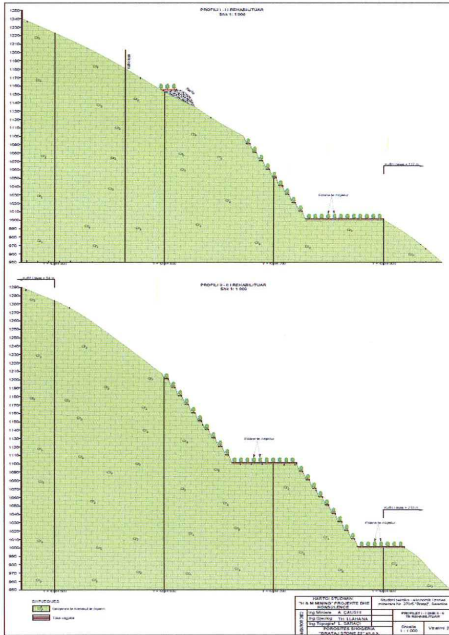
Profilet I-I dhe II-II te rehabilituar
