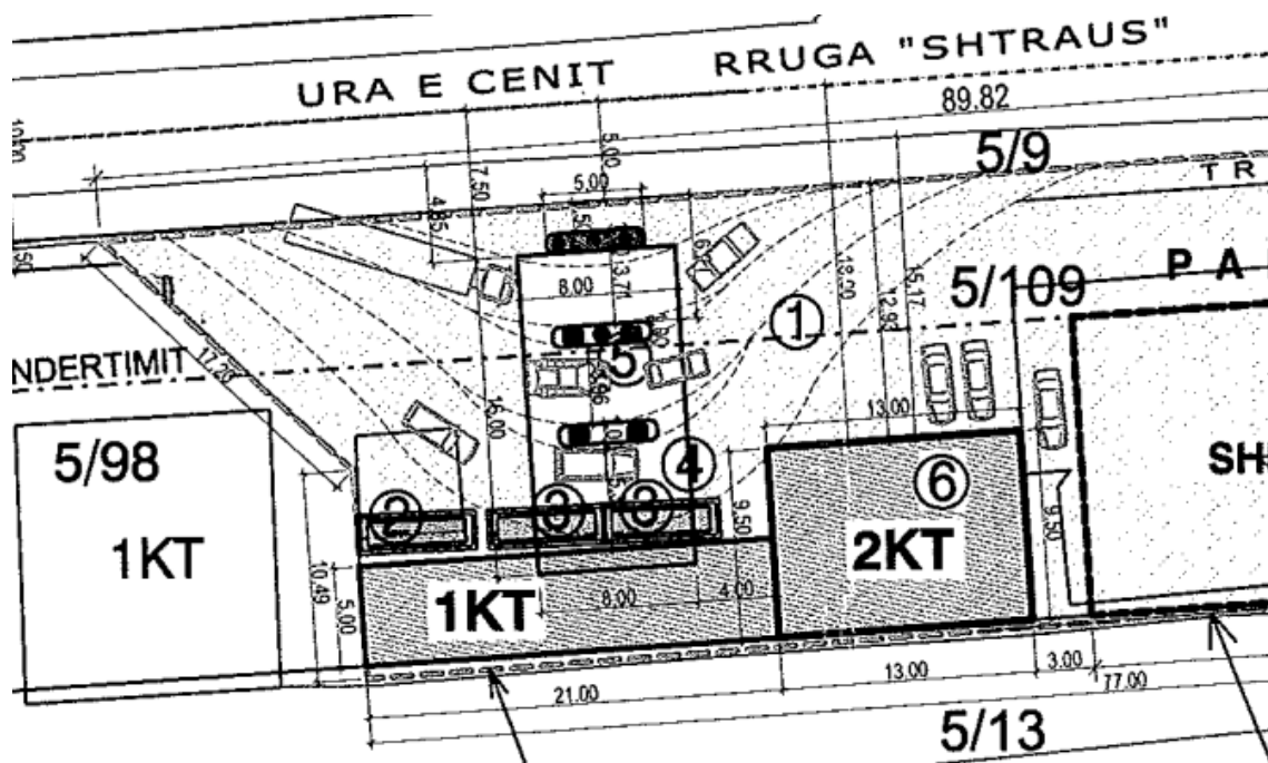
Fig.. Paraqitja skematike e menyes se funksionimit te karburantit
