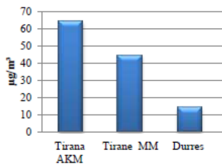
Grafiku nr 2.: Vlerat mesatare vjetore të PM10
