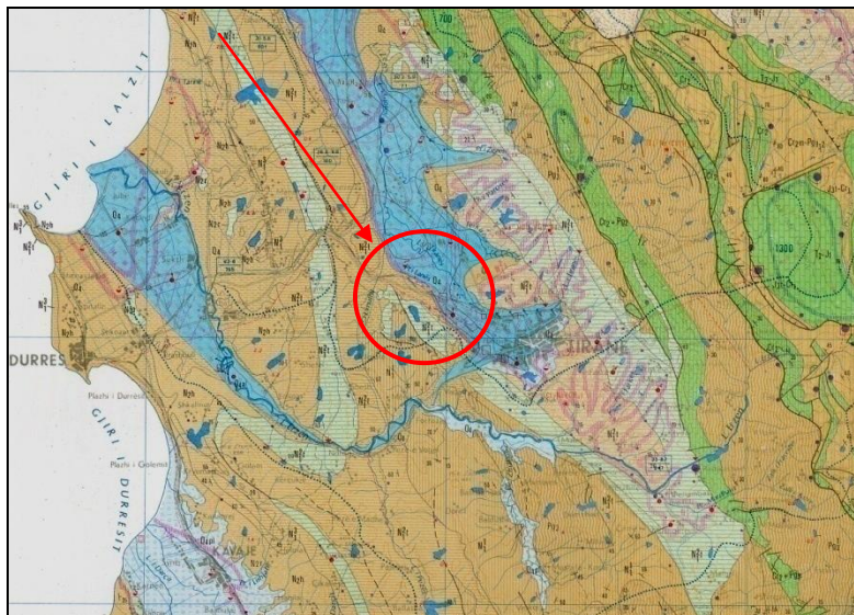
Fig. 11 Harta hidrogjeologjike e rajonit ne studim
