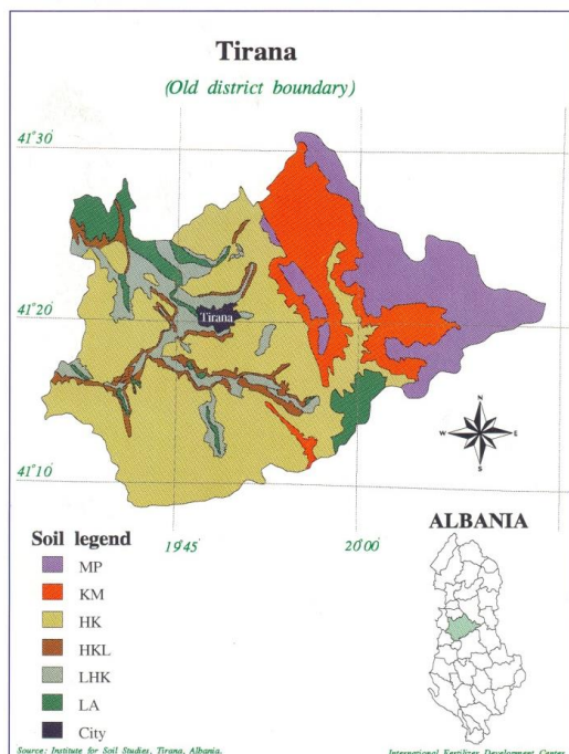
Fig.7- Harta pedologjike e rajonit
