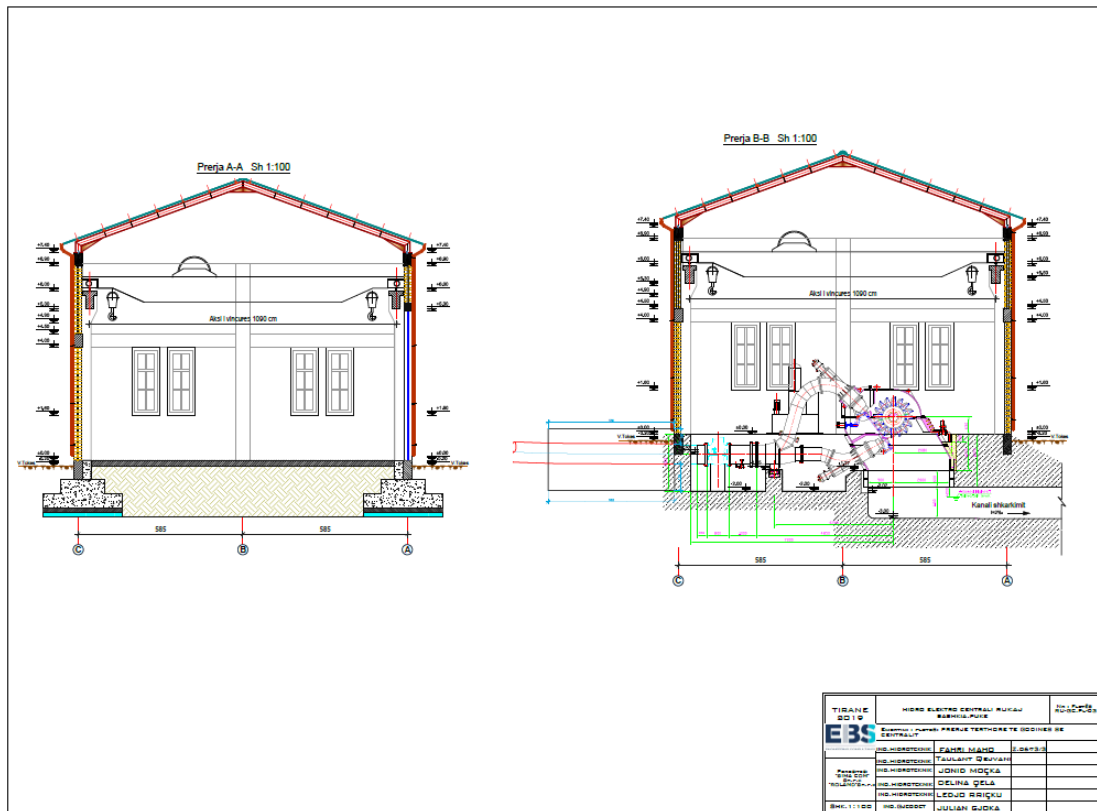
Figura 5: Prerja A-A dhe B_B e godines
