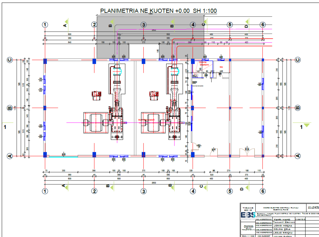
Figura 3: Planimetria e godines
