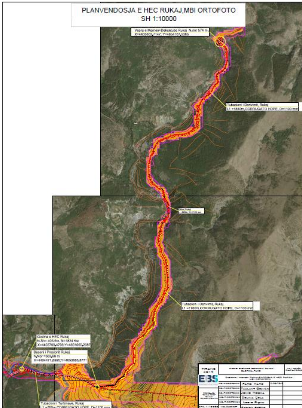
Figura 2: Planimetria e vendosjes se Hec Rukaj
