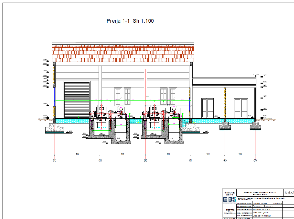
Figura 4: Prerja 1-1 e godines
