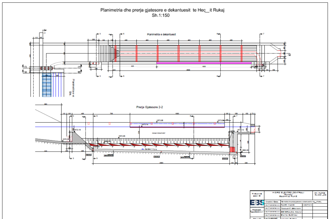
Figura 7: Planimetria dhe prerja gjatesore e dekantuesit
