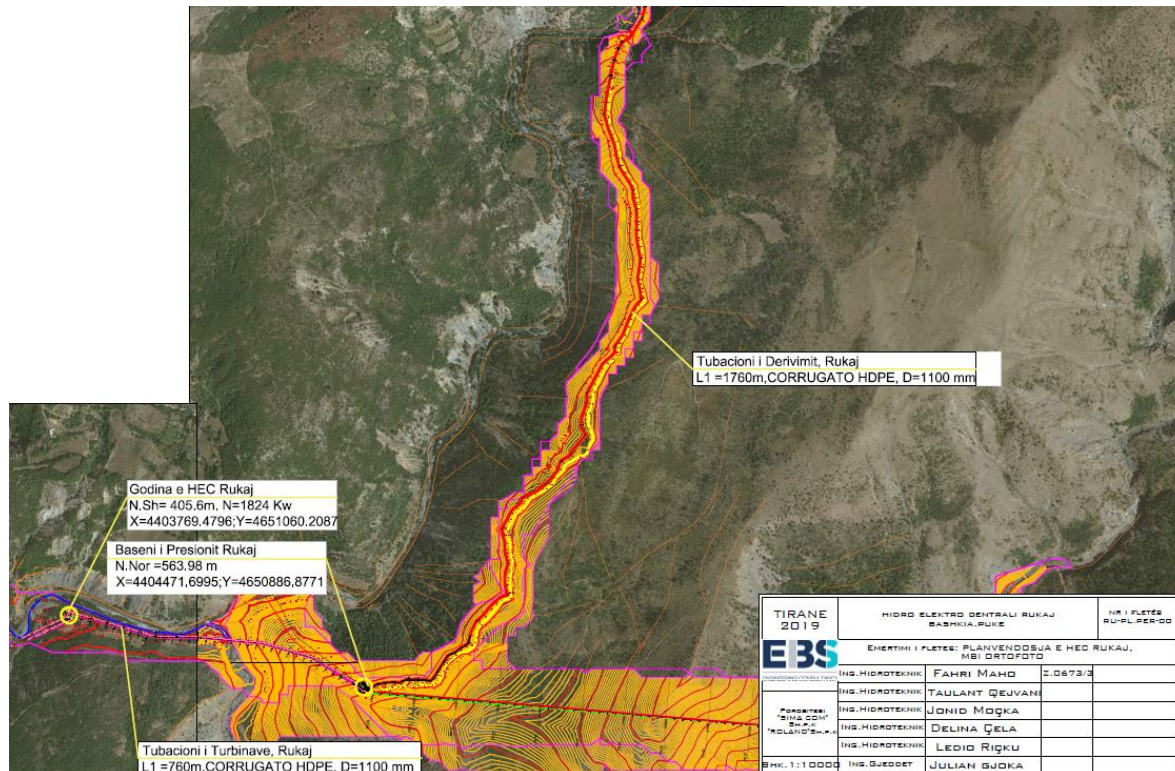
Figura 1: Planimetria e Pergjithshme e vendosjes se veprave te Hec RUKAJ me koordinata , (vendosur bashkengjitur raportit ne format A3)
