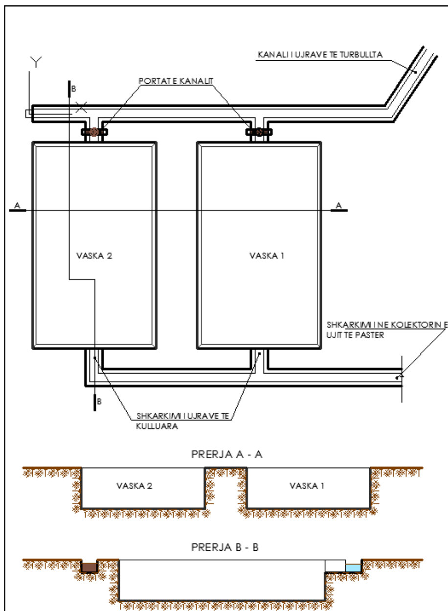
Skica e vaskave te dekantimit
