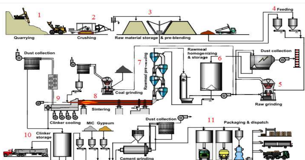
Figura. Procesi i prodhimit te Çimentos
