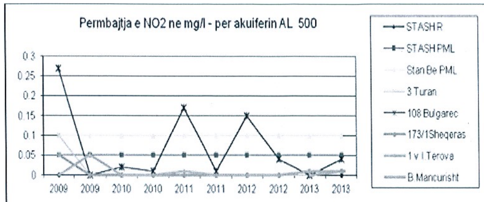
Fig- NO 2 per akuiferin AL 500
