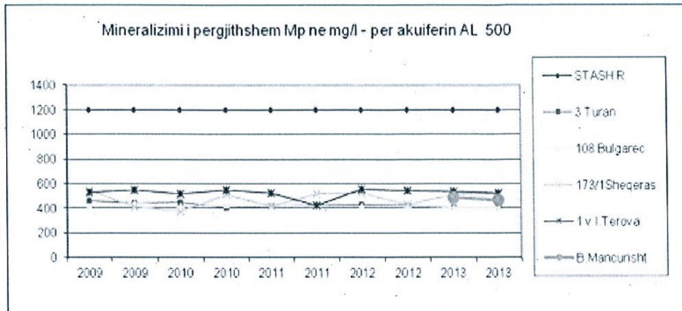
Grafiku 3 Mp per akuiferi. AL 500
