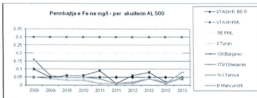
Fig- Fe per akuiferin AL 500
