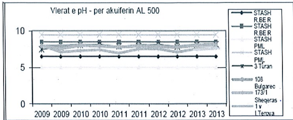
Grafiku 1 pH per akiferin AL 500
