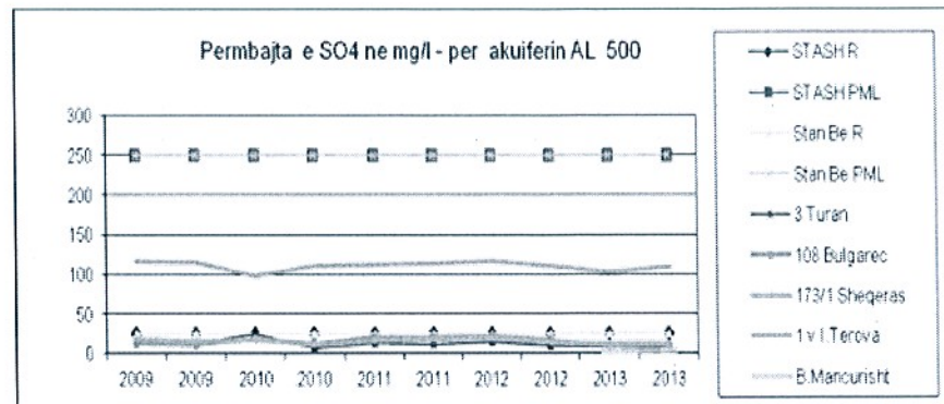
Fig.- SO4 per akuiferin AL 500
