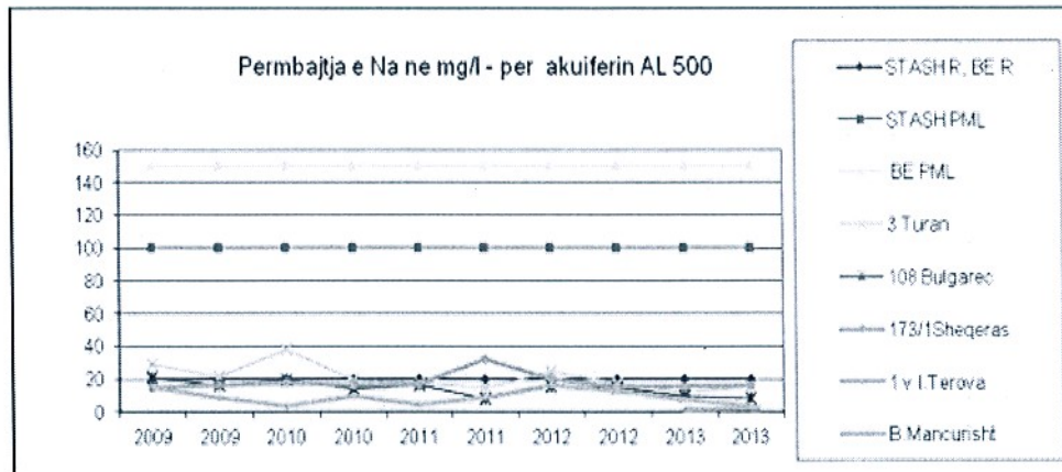
Grafiku 4 Na per akuiferin AL 500
