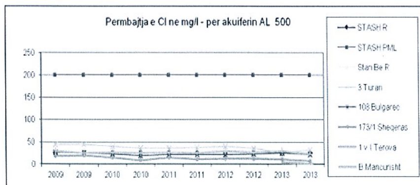
Fig.- Cl per akuiferin AL 500
