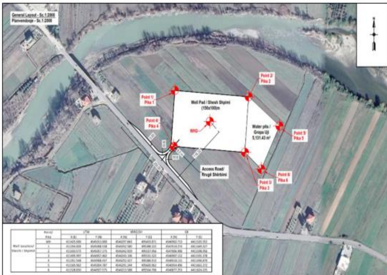
Figura 10: Planvendosja e përgjithshme e projektit. Burimi: Eni
