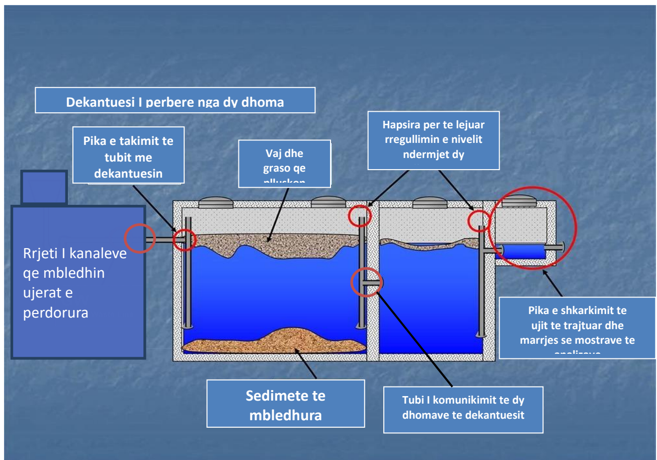
Figura 6. Skica e impjantit te trajtimit te ujerave te perdorura
