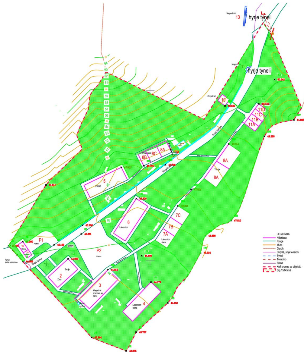
Planimetria e vendosjes se objekteve te fabrikes sipas menyres se funksionimit te procesit te prodhimit
